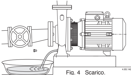
Fig. 4 Scarico.
