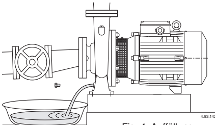
Fig. 4 Auffüllung.
