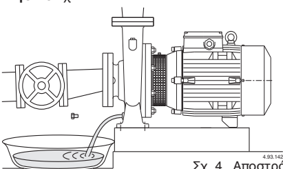
Σχ. 4 Αποστράγγιση
