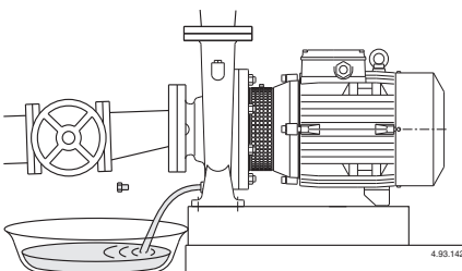
Рис. 4 Слив воды
