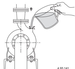
Σχ. 3 Πλήρωση
